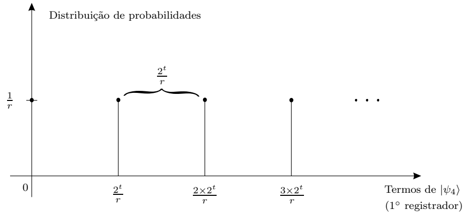
Figura 4.4: Distribuição de probabilidades de |\psi_4\rangle medida na base computacional. O eixo horizontal tem 2^t pontos; apenas os termos não nulos são mostrados. O número de picos é r e o período é 2^t/r .
